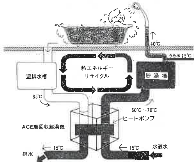
熱回収給湯機「ホットマイザー」による給湯システム
